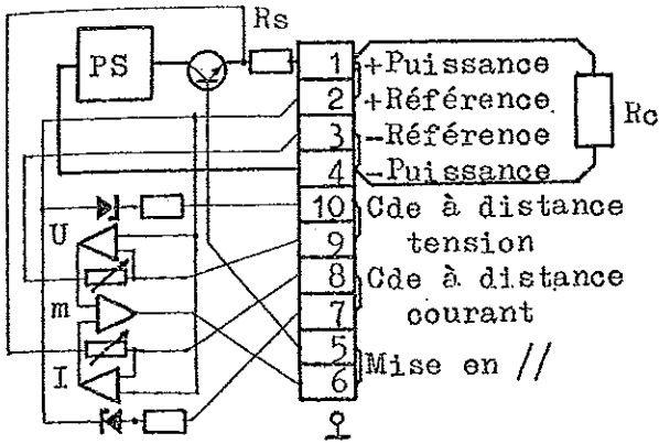
fig. 1 - schéma fonctionnel et utilisation "locale"
