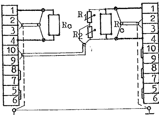
fig. 5 - Commande par une tension
