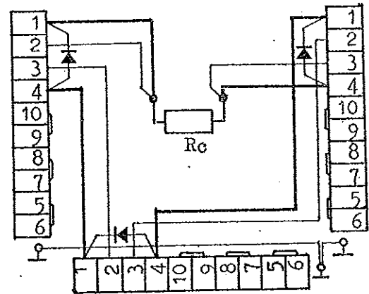
fig. 4 - Mise en série
