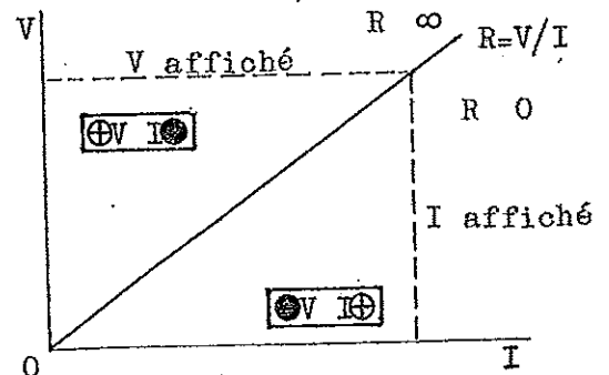
fig. 4 - Mise en série
