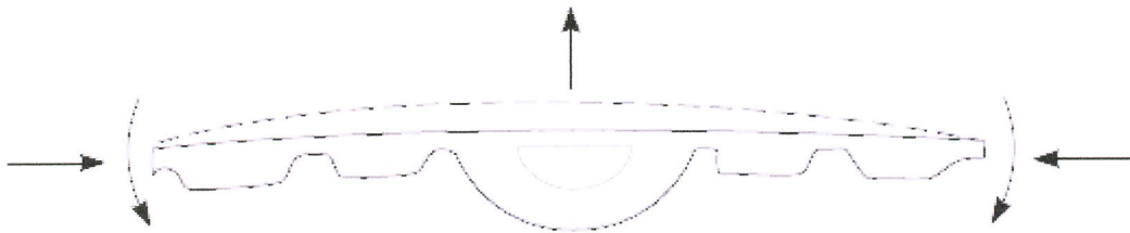
Fig. 1b Couple exercé par le bord épais sur la partie médiane mince lors du refroidissement.
