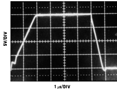
LF356
