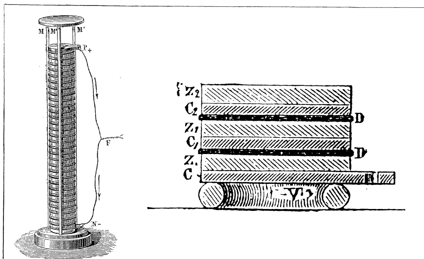
Schéma d'une pile volta en 1874.
